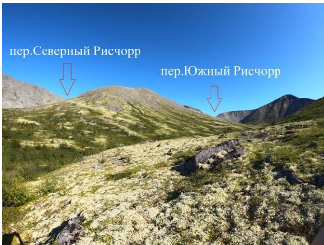
Рис.1.3 Долина р.Рисйок
