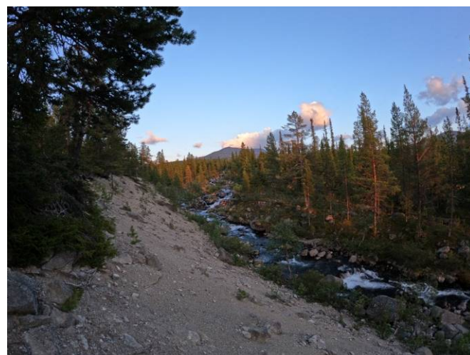
Рис.7.24 Долина р.Часнайок
